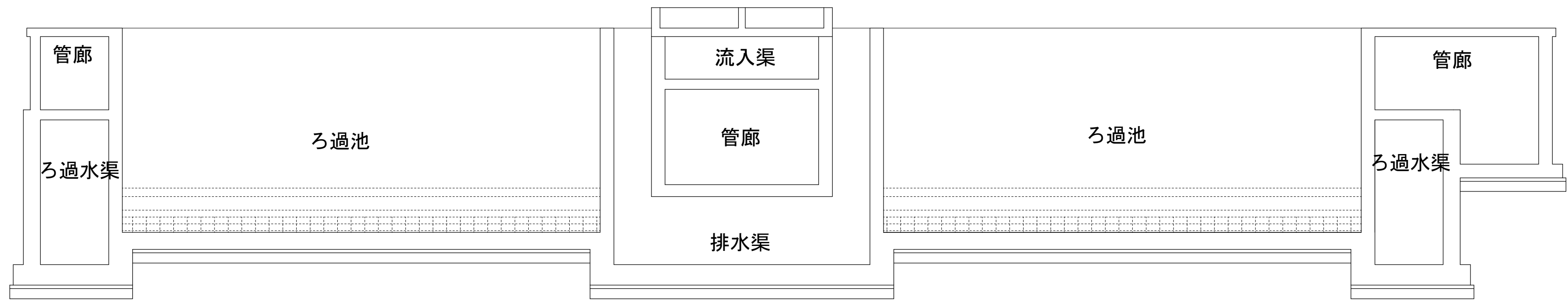
C－C' 断面
