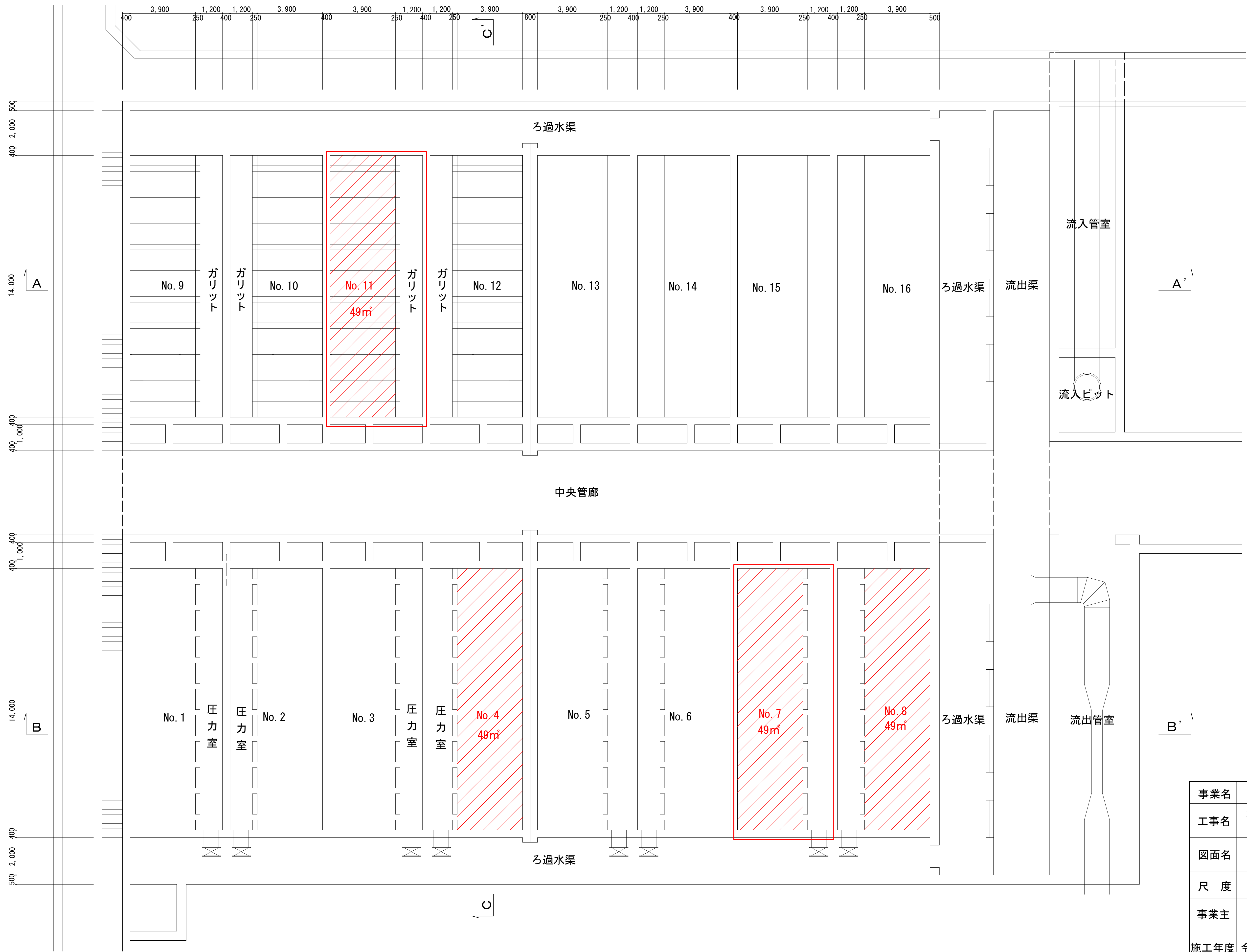
平 面 図
